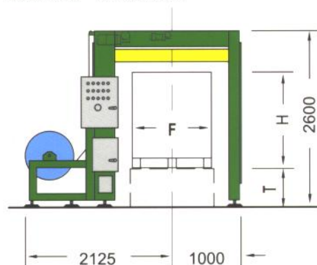
Vista laterale - Lateral view Vista lateral - Seitenansicht
